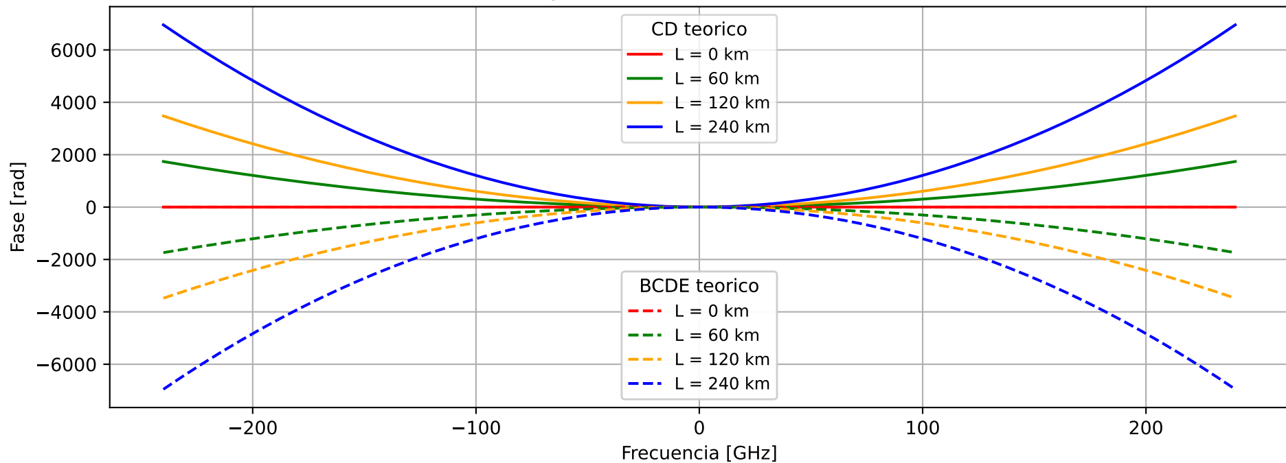
Respuesta de Fase. BR = 120 GBd
